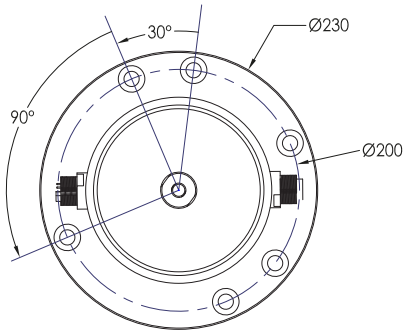
Croquis de la versión en aluminio.
