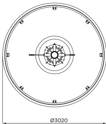
Ejemplo MBM30
